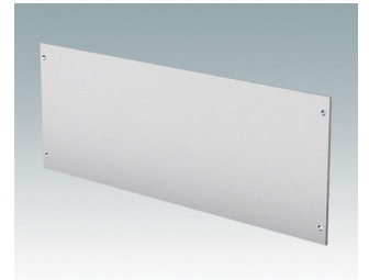
M6400702 Plaque avant 210 Aluminium Anodisé mat 247x2x90,8mm
