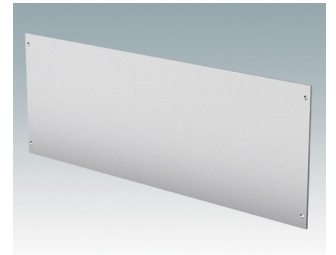
M6400706 Plaque avant 312 Aluminium Anodisé mat 322x2x115,8mm
