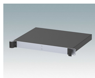
M6219129 COMBIMET 19" 1Ux365mm panneau supérieur plein Aluminium Noir RAL 9005 43,6x482,6x365mm
