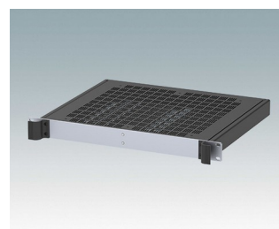
M6219169 COMBIMET 19" 1Ux365mm avec aération Aluminium Noir RAL 9005 43,6x482,6x365mm
