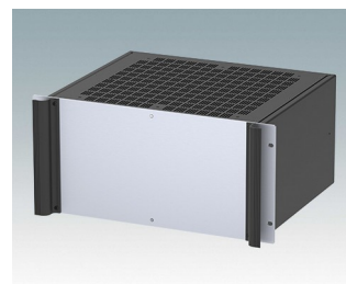
M6219569 COMBIMET 19" 5Ux365mm avec aération Aluminium Noir RAL 9005 221x482,6x365mm
