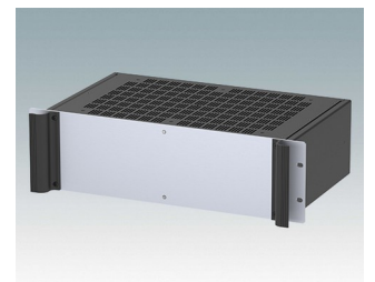
M6219349 COMBIMET 19" 3Ux265mm avec aération Aluminium Noir RAL 9005 132,5x482,6x265mm
