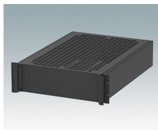
M6219389 COMBIMET 19" 3Ux610mm avec aération Aluminium Noir RAL 9005 132,5x482,6x609,6mm
