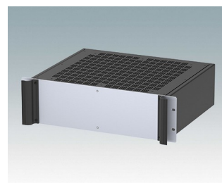
M6219369 COMBIMET 19" 3Ux365mm avec aération Aluminium Noir RAL 9005 132,5x482,6x365mm
