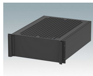
M6219489 COMBIMET 19" 4Ux610mm avec aération Aluminium Noir RAL 9005 177x482,6x609,6mm
